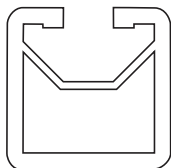
14005 Size: 1 X 1 X .100 Wt. Lin. Ft. .442
