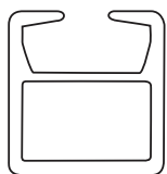
14000 Size: 1 X 1 X .093 Wt. Lin. Ft. .398
