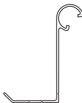
14055 Female Awning Size: 27' Wt. Lin. Ft. .385
